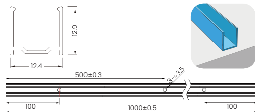
Aluminum Profile : 1213
