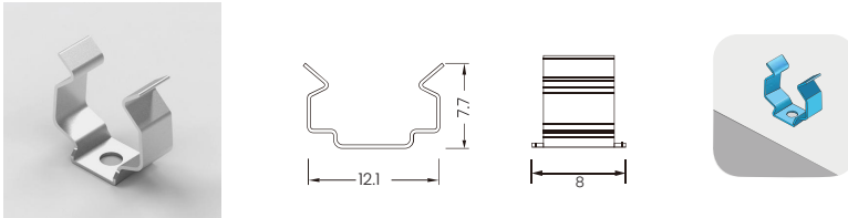
Aluminum Profile : 1213
